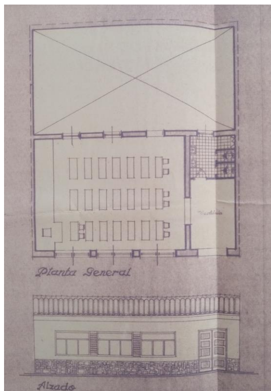
Plano de la planta general y alzado de la escuela
