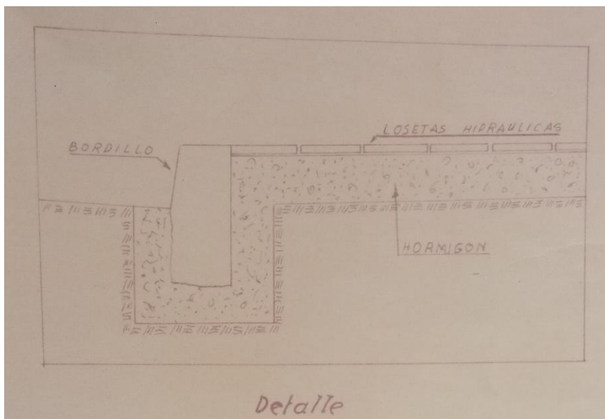
Plano detalle de la construcción de la acera
